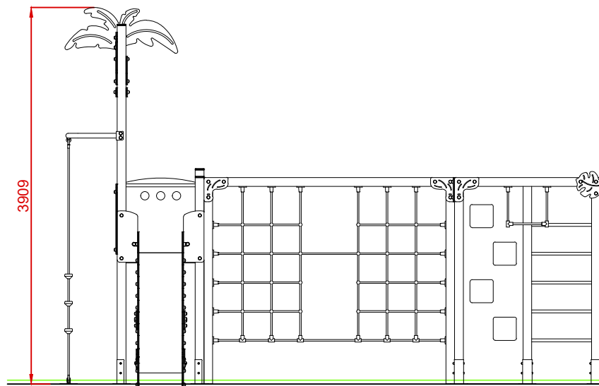
ALZADO
