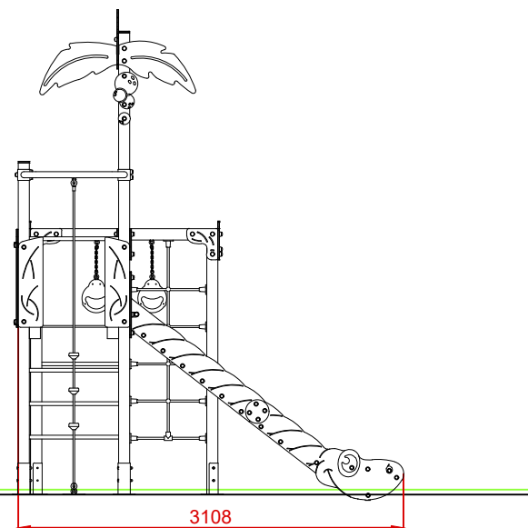
PERFIL IZQUIERDO
