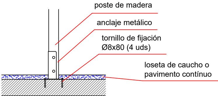
ESQUEMA DE CIMENTACIÓN EN HORMIGÓN E: 2/1
