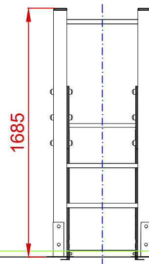
PERFIL IZQUIERDO
