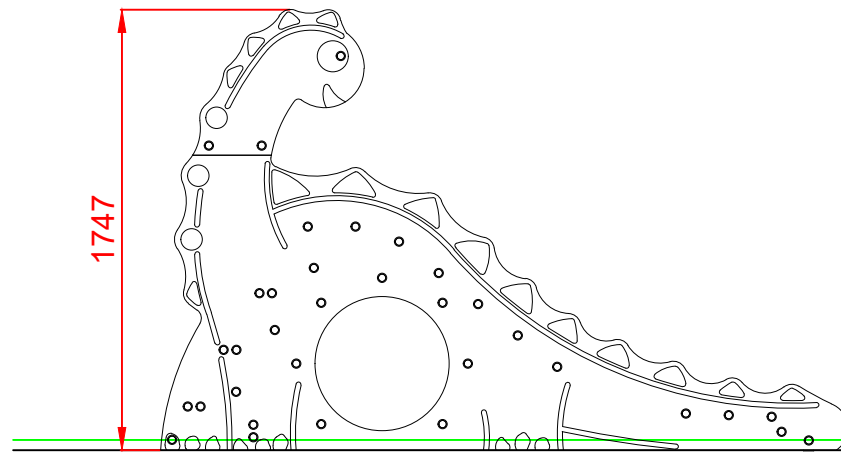
ALZADO
