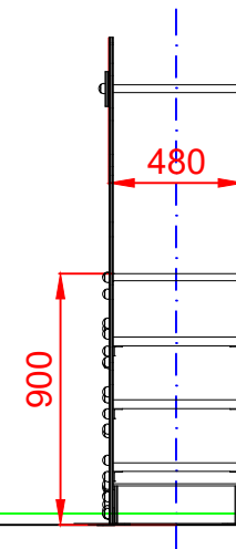
PERFIL IZQUIERDO
