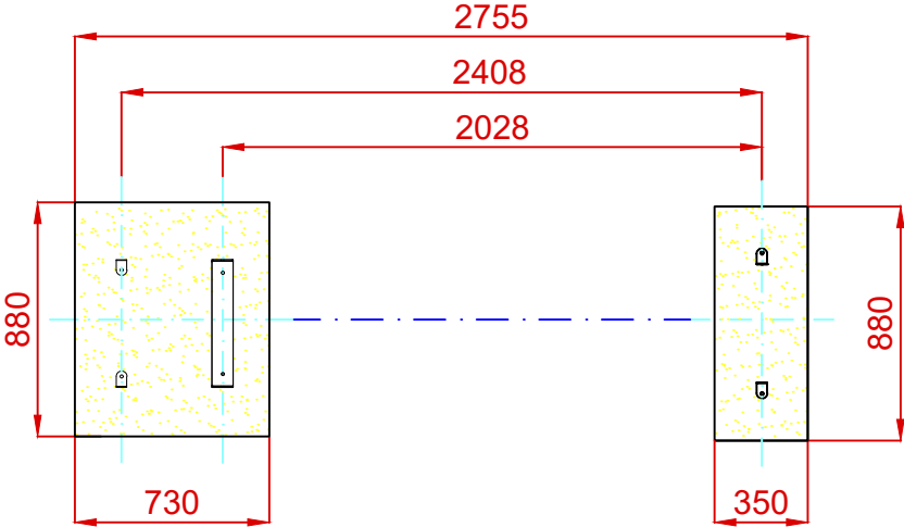
PLANTA CIMENTACIÓN
