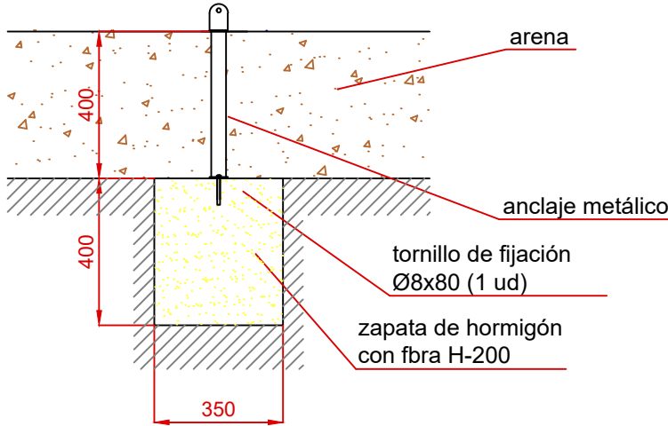
ESQUEMA DE CIMENTACIÓN EN HORMIGÓN E: 2/1
