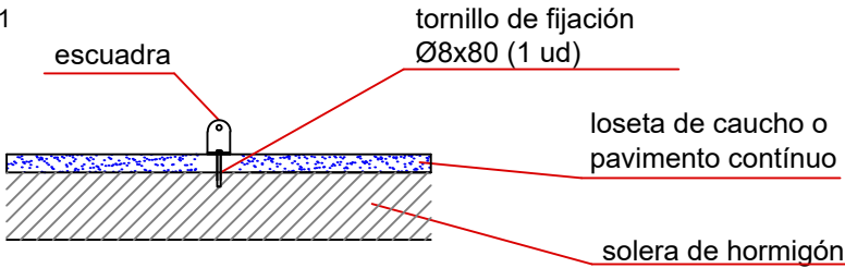
ESQUEMA DE CIMENTACIÓN EN HORMIGÓN E: 2/1
