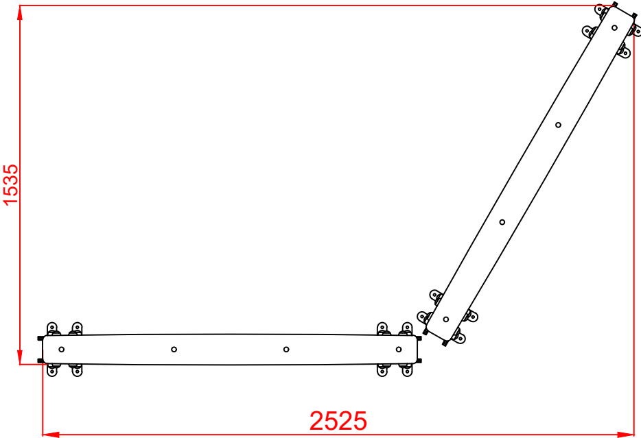
PLANTA
