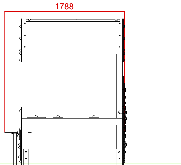
PERFIL
