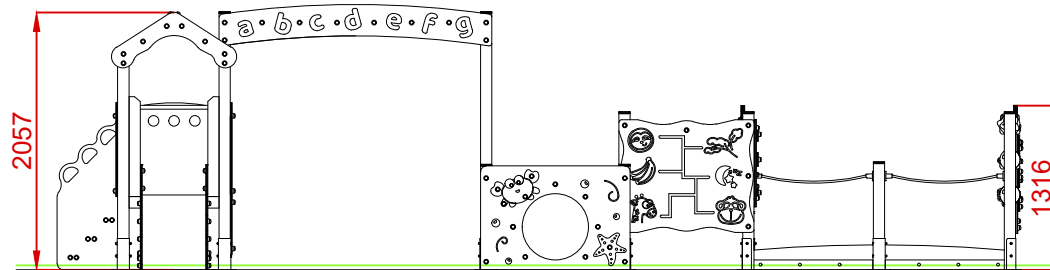
ALZADO
