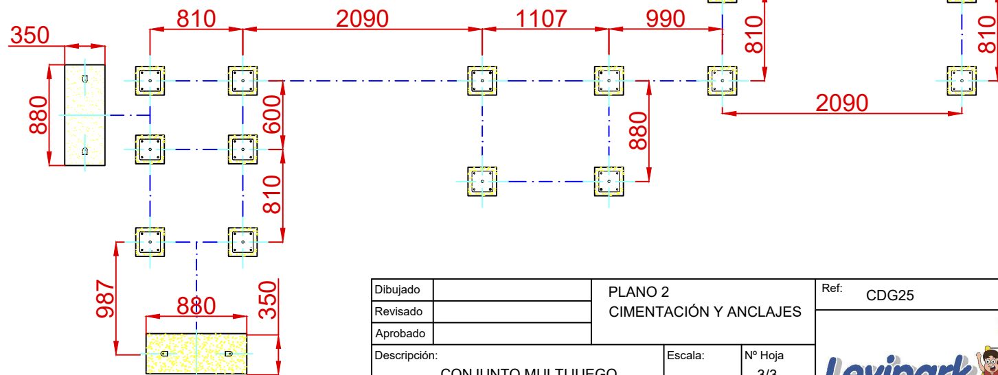
PLANTA CIMENTACIÓN
