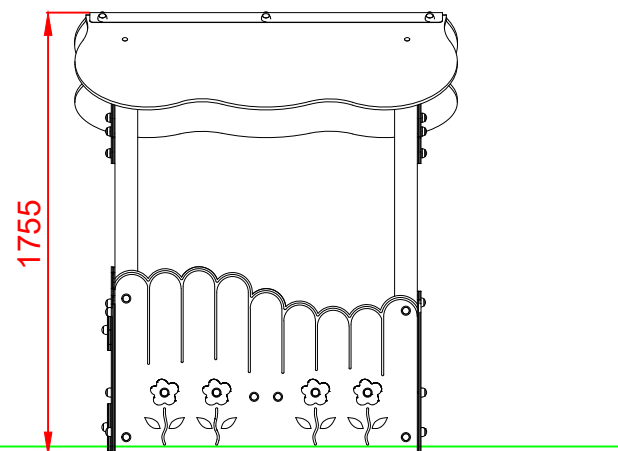
PERFIL IZQUIERDO
