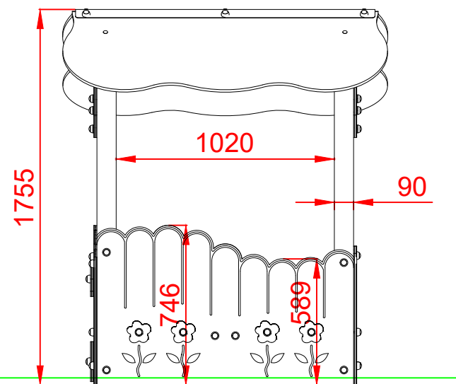
PERFIL IZQUIERDO
