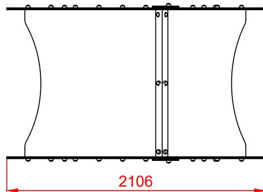
PLANTA
