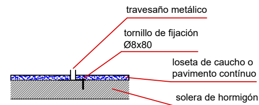
ESQUEMA DE CIMENTACIÓN EN HORMIGÓN
