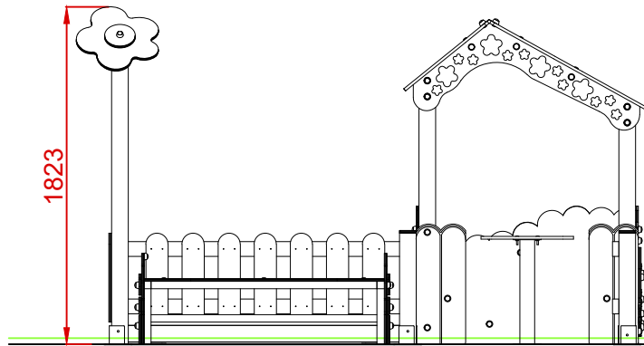
ALZADO
