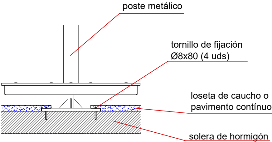
ESQUEMA DE CIMENTACIÓN EN HORMIGÓN
