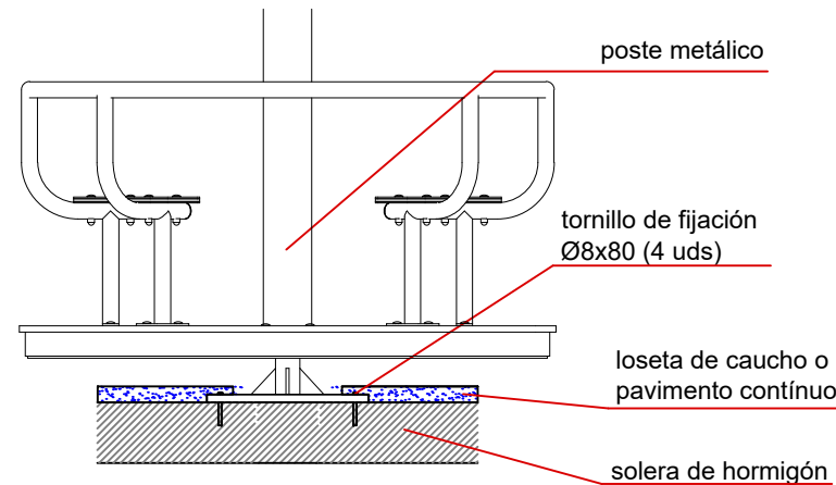
ESQUEMA DE CIMENTACIÓN EN HORMIGÓN
