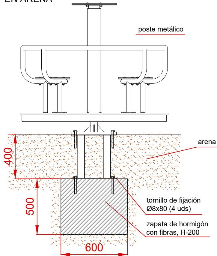
ESQUEMA DE CIMENTACIÓN EN ARENA
