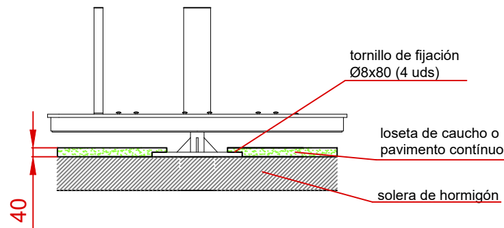
ESQUEMA DE CIMENTACIÓN EN HORMIGÓN VERSIÓN 1
