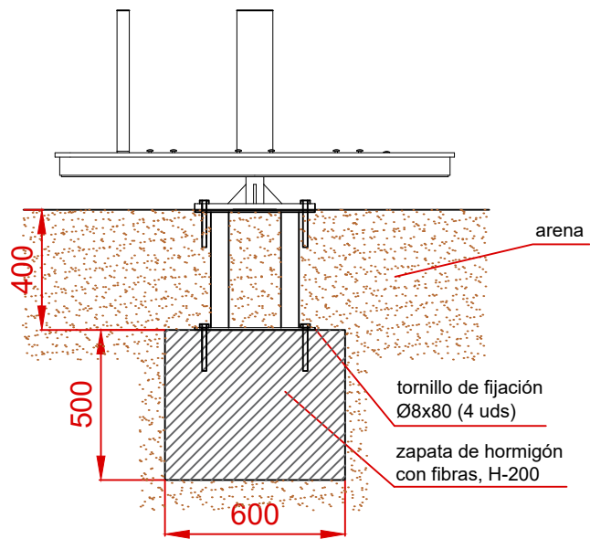
ESQUEMA DE CIMENTACIÓN EN ARENA
