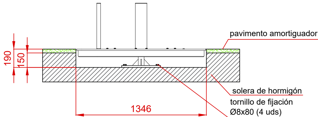
ESQUEMA DE CIMENTACIÓN EN HORMIGÓN VERSIÓN 2
