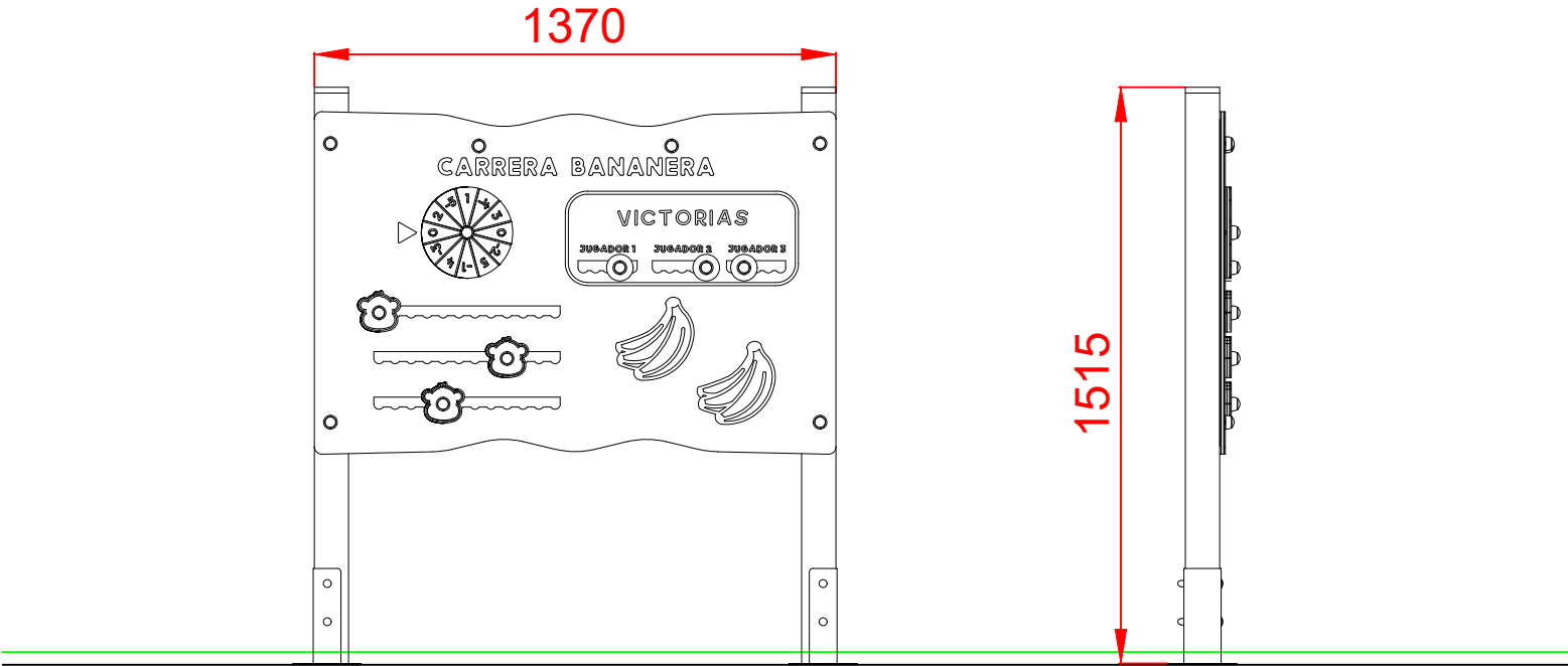
ALZADO
