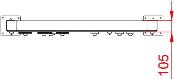
PLANTA
