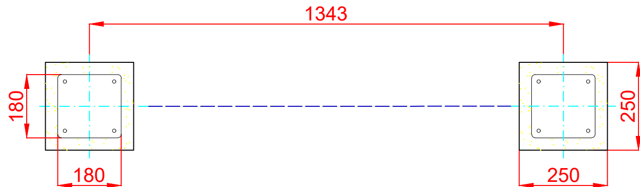
PLANTA CIMENTACIÓN E: 2/1
